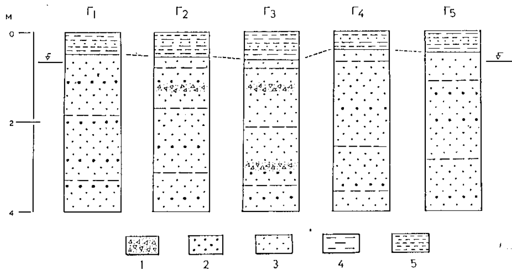
Εικ. 10. Λιθολογικές στήλες των γεωτρήσεων Γ1-Γ5. (1. Χαλίκες 2. Μέση, Χονδρόκοκκος άμμος 3. Λεπτή άμμος, 4. Ιλύς, 5. Αργίλος).
